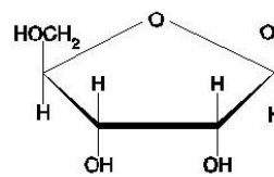
Ribose
