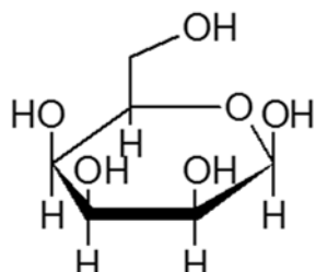
\beta -D-Talopyranose
