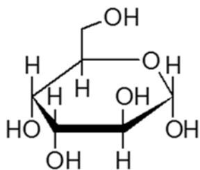
\alpha -D-Altropyranose
