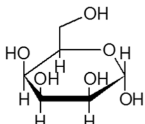
\alpha -D-Talopyranose
