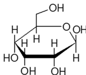
\beta -D-Allopyranose
