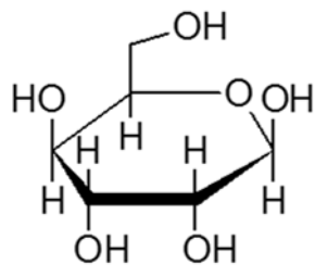
\beta -D-Gulopyranose
