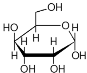
\alpha -D-Gulopyranose
