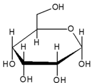
\alpha -D-Allopyranose
